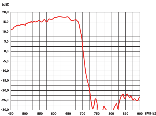
Curva de ganancia Diamond
